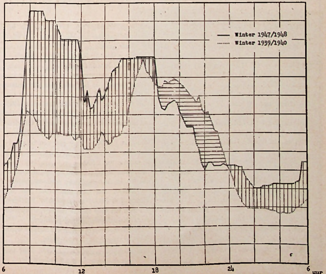
Dagbelastingkromme van de Rotterdamse centrale
